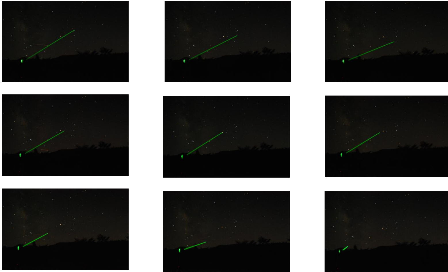
さそり座を構成する星の順次ポインティングの様子
